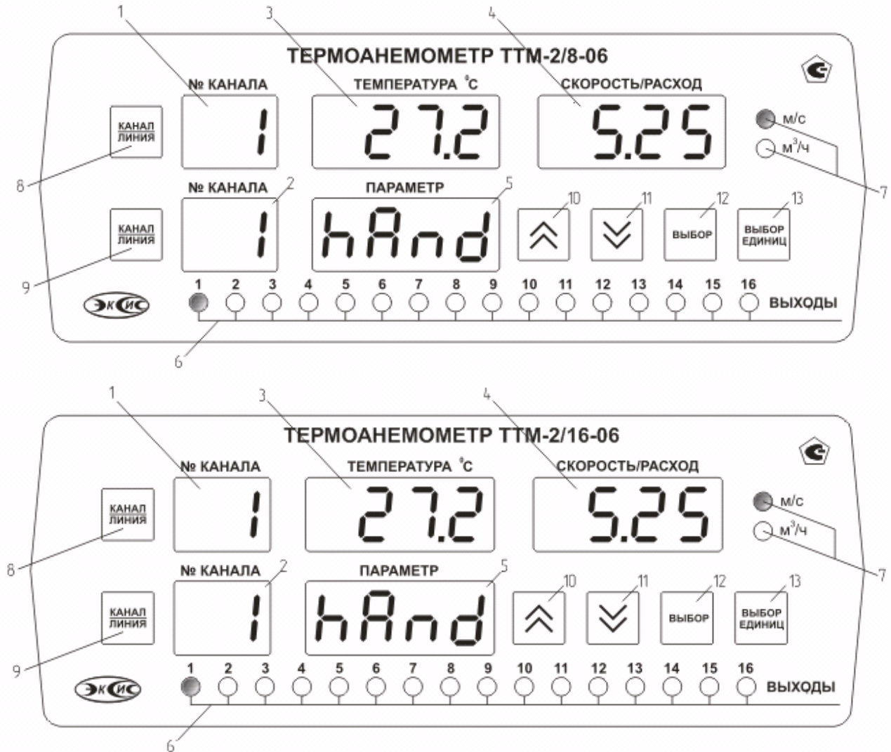
Рисунок 3.1 Вид лицевой панели прибора, сверху вниз исполнение: TTM-2/8-06, TTM-2/16-06
