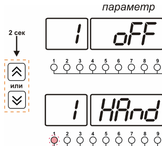
Рисунок 6.5 Ручное включение исполнительного устройства первого канала управления
