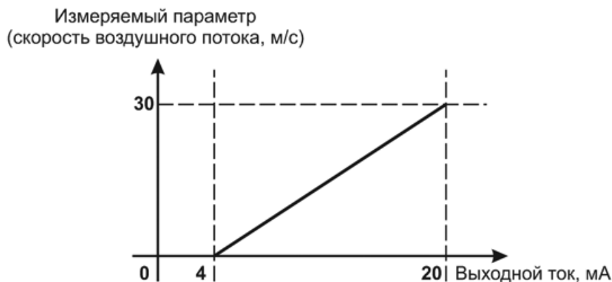
Рисунок 3.14 Пределы измерения скорости воздушного потока и выходной ток
